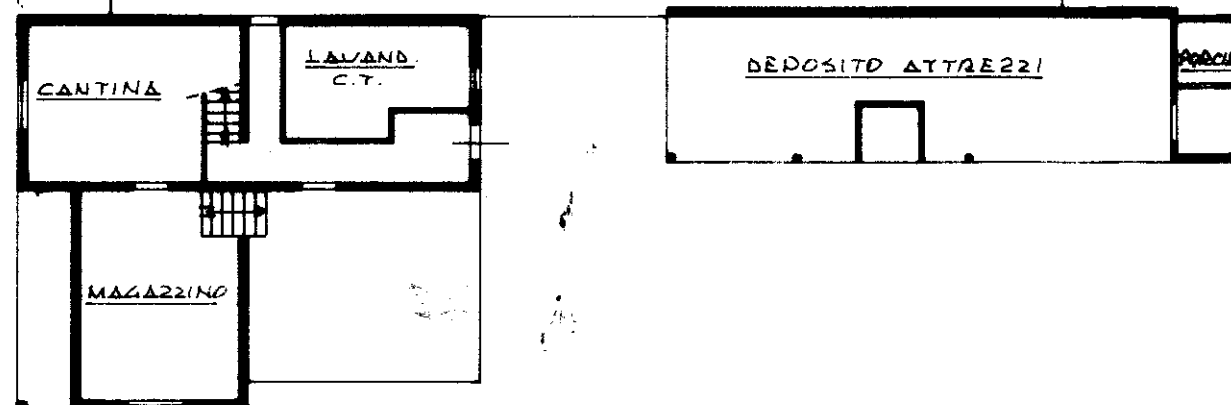
PIANO TERRA - H. 2.20
